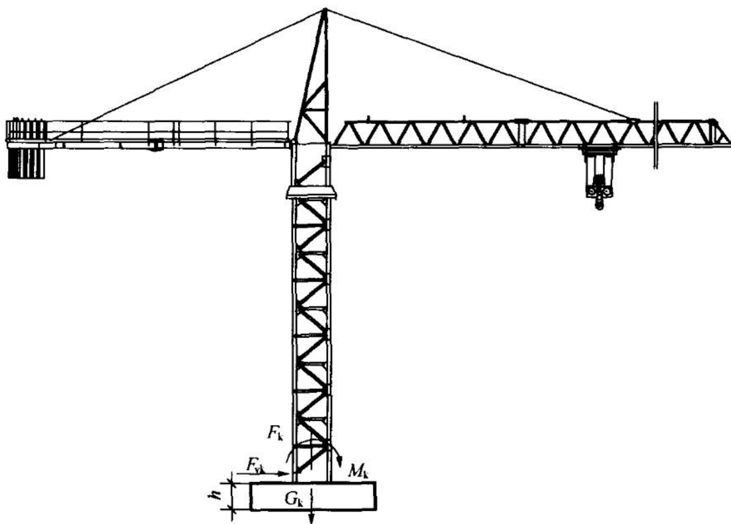
图 3.2.3 塔式起重机板式基础计算简图
