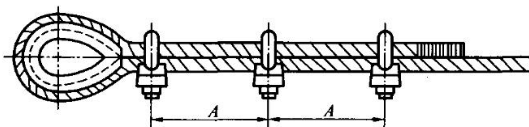
图 6.2.4 钢丝绳夹压板布置图
