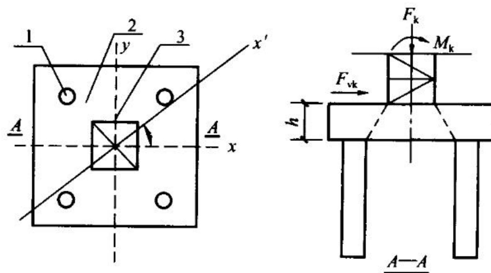
图 3.2.4 塔式起重机方形承台桩基础
